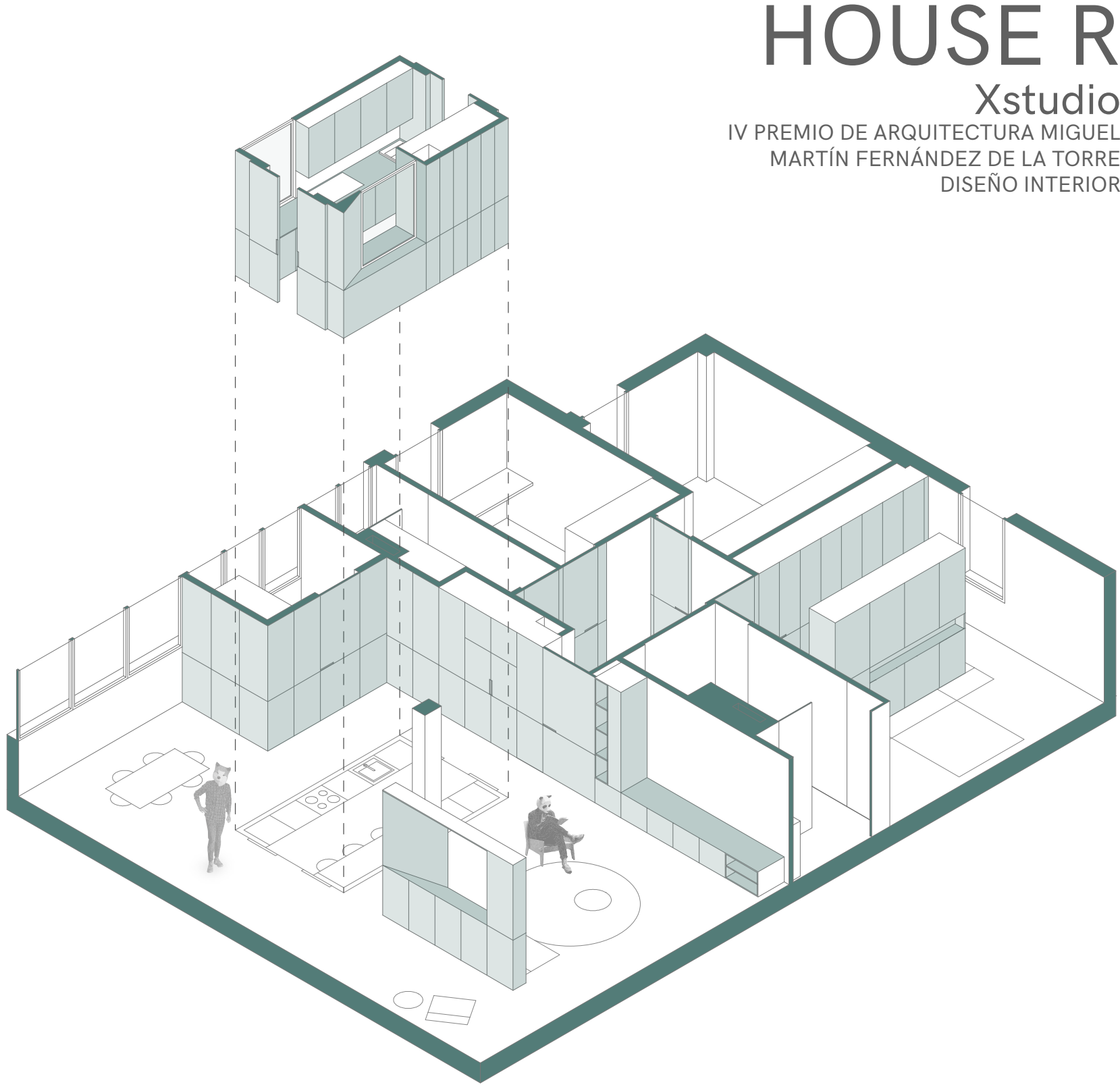
ESQUEMA AXONOMÉTRICO
