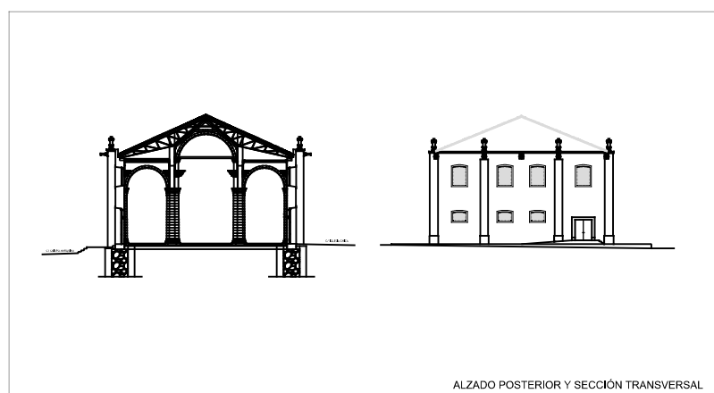
ALZADO POSTERIOR Y SECCIÓN TRANSVERSAL
