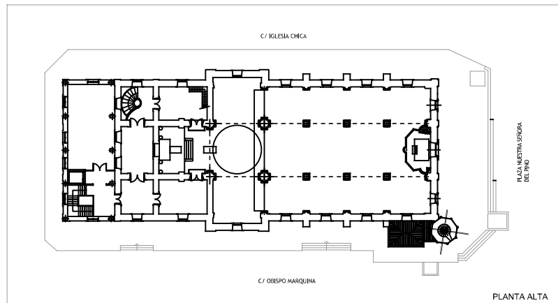
PLANTA ALTA
