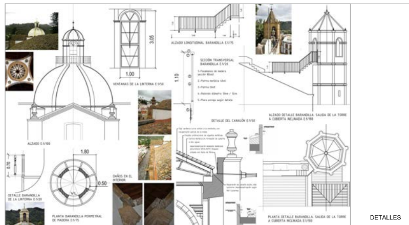
DETALLES
