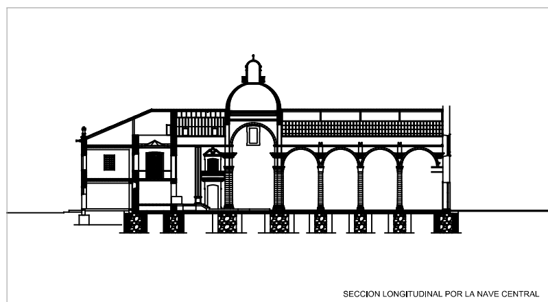
SECCIÓN LONGITUDINAL POR LA NAVE CENTRAL
